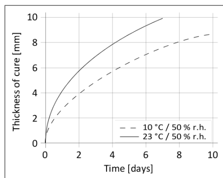
Diagram 1: Vitesse de polymérisation du Sikaflex®-290 DC PRO
