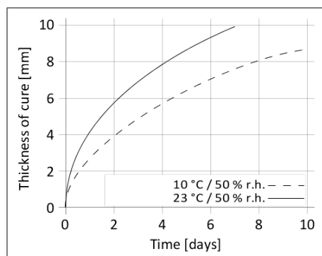
Grafico 1: Velocità di polimerizzazione per SikaTack® DRIVE (Purform®)
