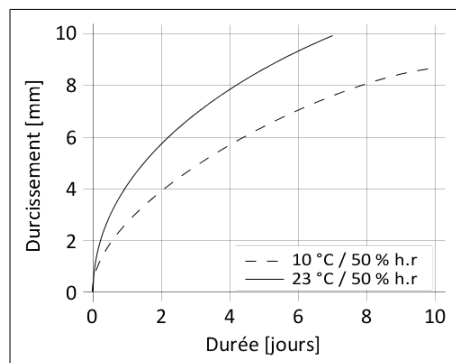
Diagramme 1 : Vitesse de polymérisation du Sikaflex®-223
