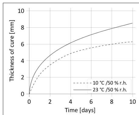
Diagram 1: Rychlost vytvrzení Sikaflex®-552 AT
