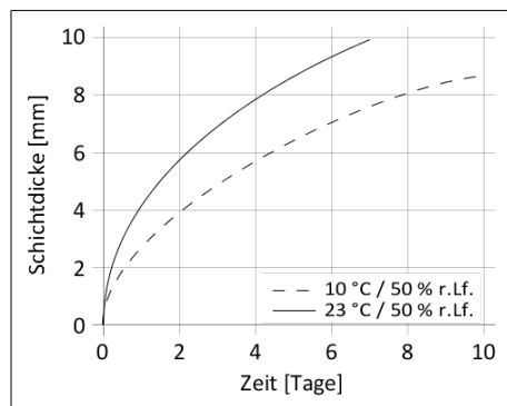
Diagramm 1: Durchhärtegeschwindigkeit von Sikaflex®-223
